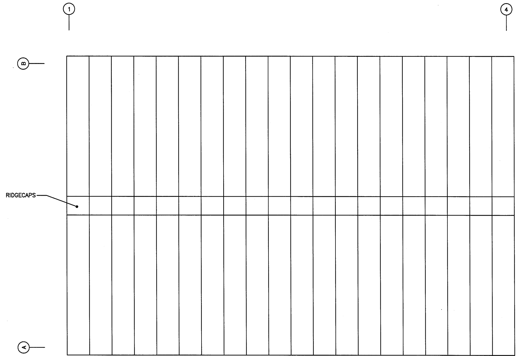
ROOF SHEETING PLAN N.T.S.
