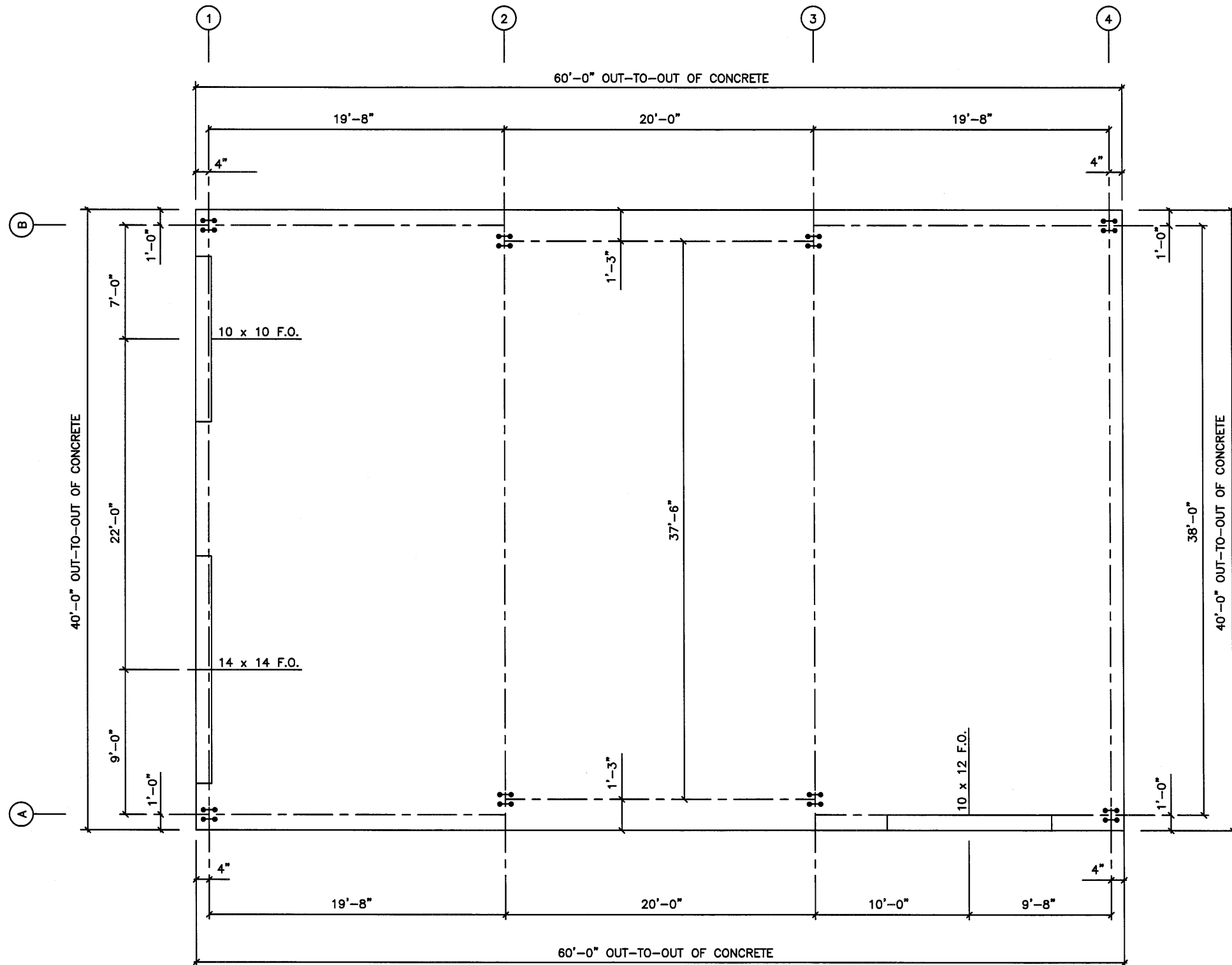
ANCHOR BOLT PLAN N.T.S.
